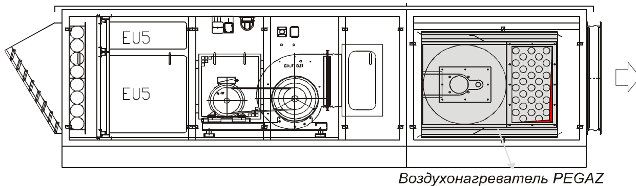
Рис. 5. Нагревательный модуль «PEGAZ», работающий в качестве подвешеного зонального нагревателя.
