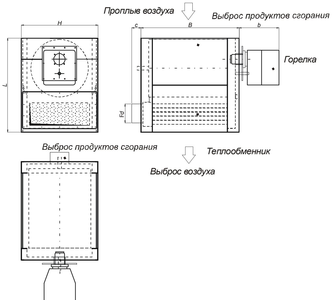
Рис.3. Воздуонагреватель PEGAZ с вертикальным пропływом воздуха
